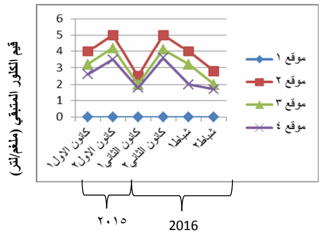
شكل رقم (٦) التغيرات النصف شهرية لقيم الكلور المتبقي في المياه للفترة من كانون الأول 2015 ولغاية شباط 2016
