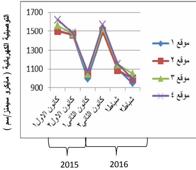
شكل رقم (٣) التغيرات النصف شهرية في قيم التوصيلية الكهربائية للفترة من كانون الأول 2015 ولغاية شباط 2016
