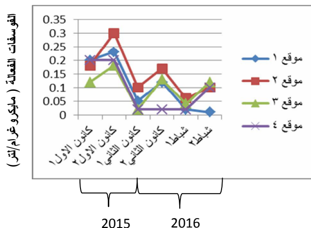
شكل رقم (٨) التغيرات النصف شهرية لقيم الفوسفات للمدة من كانون الأول 2015 ولغاية شباط 2016
