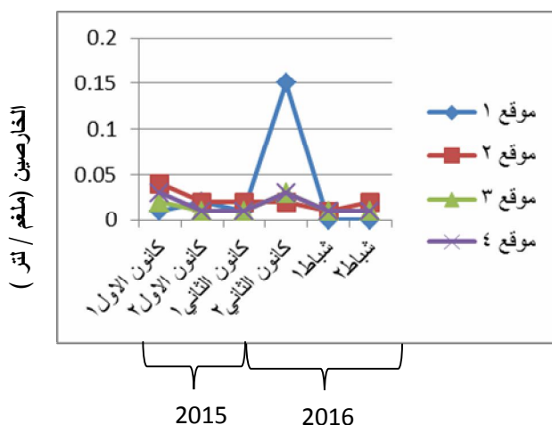
شكل رقم (١٢) التغيرات النصف شهرية لقيم الخارصين للمدة من كانون الأول 2015 ولغاية شباط 2016
