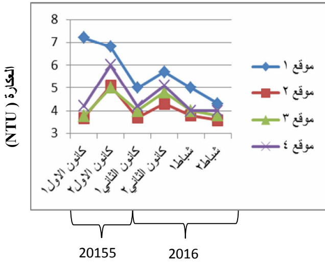
شكل رقم (٥) التغيرات النصف شهرية لعكارة الماء للفترة من كانون الأول 2015 ولغاية شباط 2016
